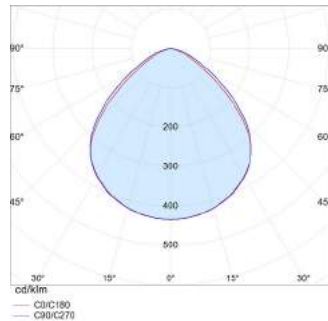
6721.408.V3.LM11 54 W SATIINIÄKRYYLII
