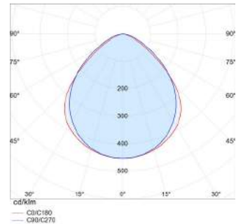
6741.408.V3.LM11 71 W SATIINIÄKRYYLII
